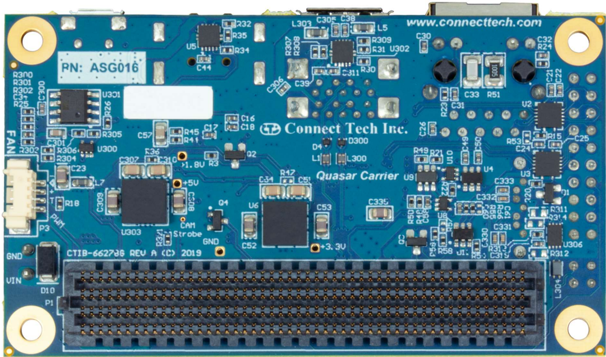
CONNECTOR FOR TX1/TX2/TX2i/TX2-4GB MODULE P1
