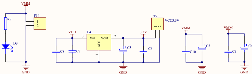
POWER_PART
