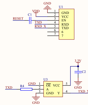
XBEE_PART
