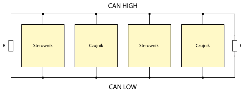
Rysunek 2. Topologia magistrali CAN
