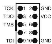
Rys. 1. Przepisanie sygnałów do styków złącza wyjściowego w trybie JTAG/IEEE532
