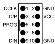
Rys. 2. Przepisanie sygnałów do styków złącza wyjściowego w trybie konfigurowania układów FPGA
