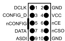
Rys. 3. Przepisanie sygnałów do styków złącza wyjściowego w trybie programowania konfiguratorów Flash
