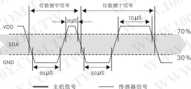
图 23: 单总线分解时序图
