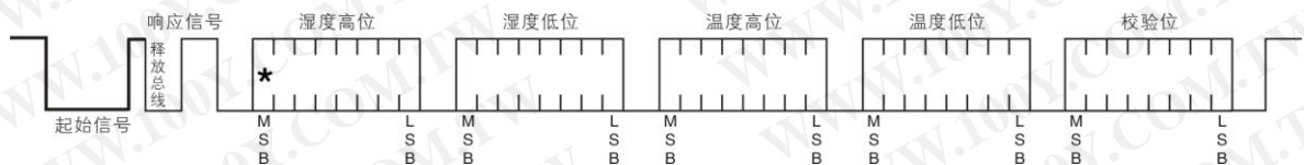
图 20： AM2321 单总线通信协议
