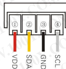
图 4: AM2321 接线图
