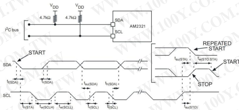
图 13: AM2321 典型的 I2C 总线应用电路和时序图
