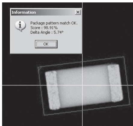
Fot. 7.5. Centrowanie podzespołów w systemie wizyjnym
