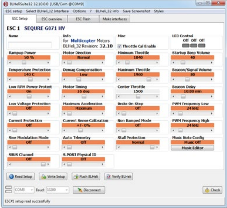
BLHeli_32固件可视化编程调参界面
