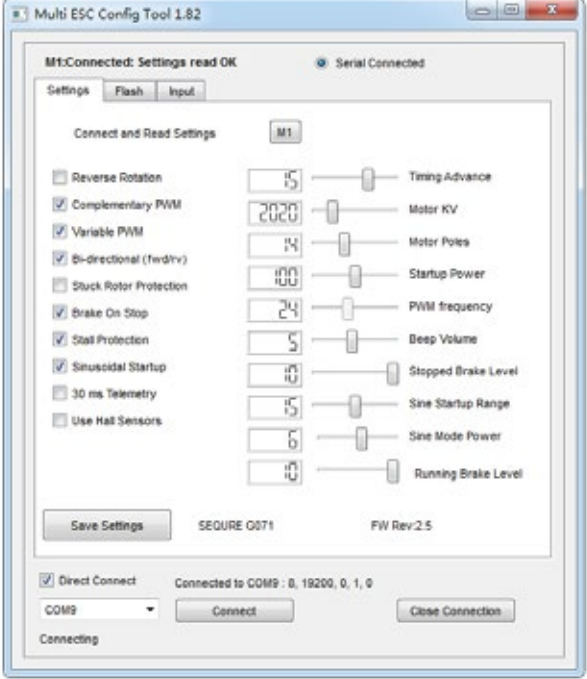
AM32固件可视化编程调参界面
