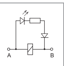
C: Opcja 3, 5, 54 LED (AC)
