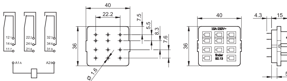
Przełącznik 62.33 wraz z gniazdem 92.13 ma wysokość 63.3 mm
