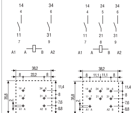
62.22-4300 R Rysunek otworów montażowych
