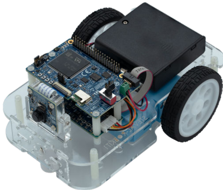
Figure 1. STEVAL-ROBKIT1
