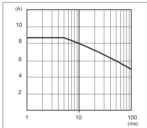
P78-5 Szczytowy prąd wyjścia w czasie (78.50)
