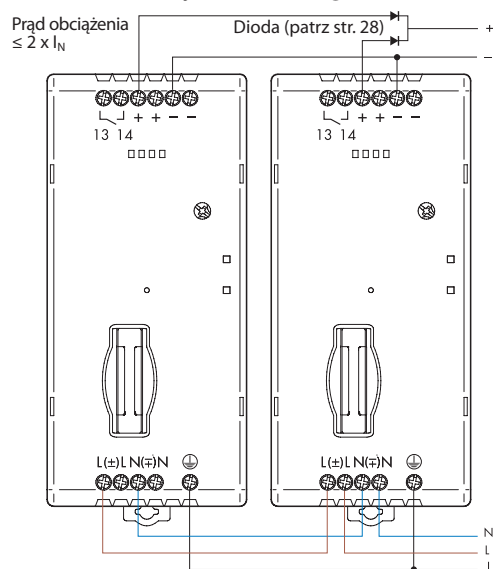
Połączenia równoległe
