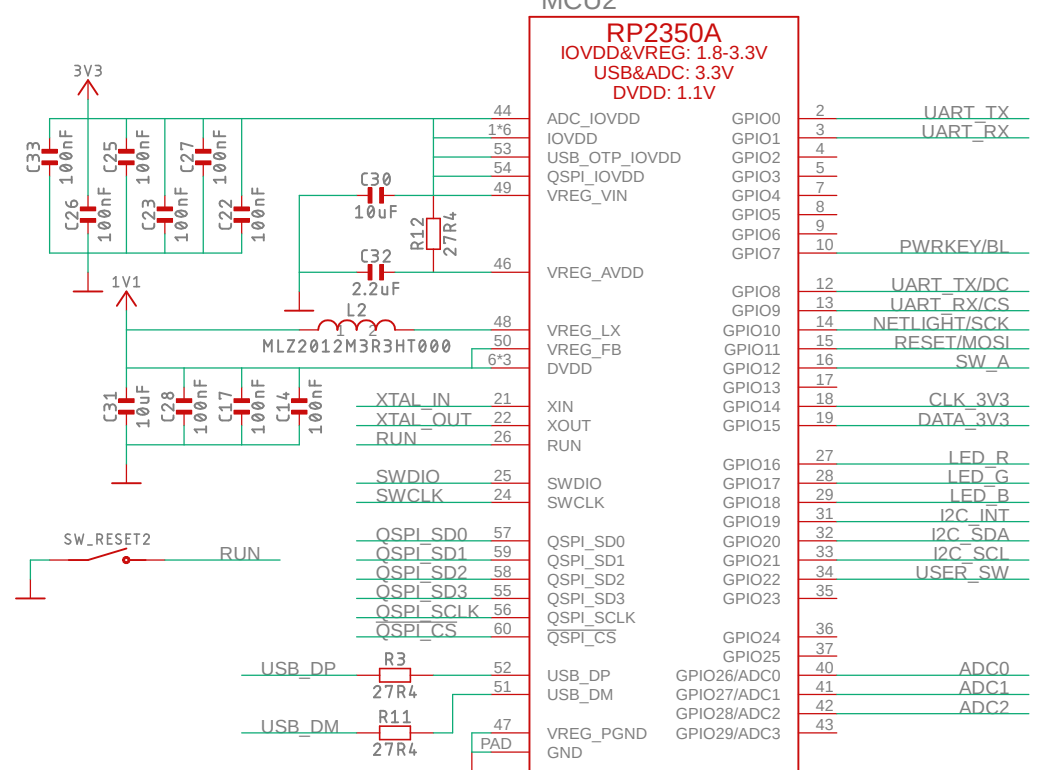
RP2350 MCU
