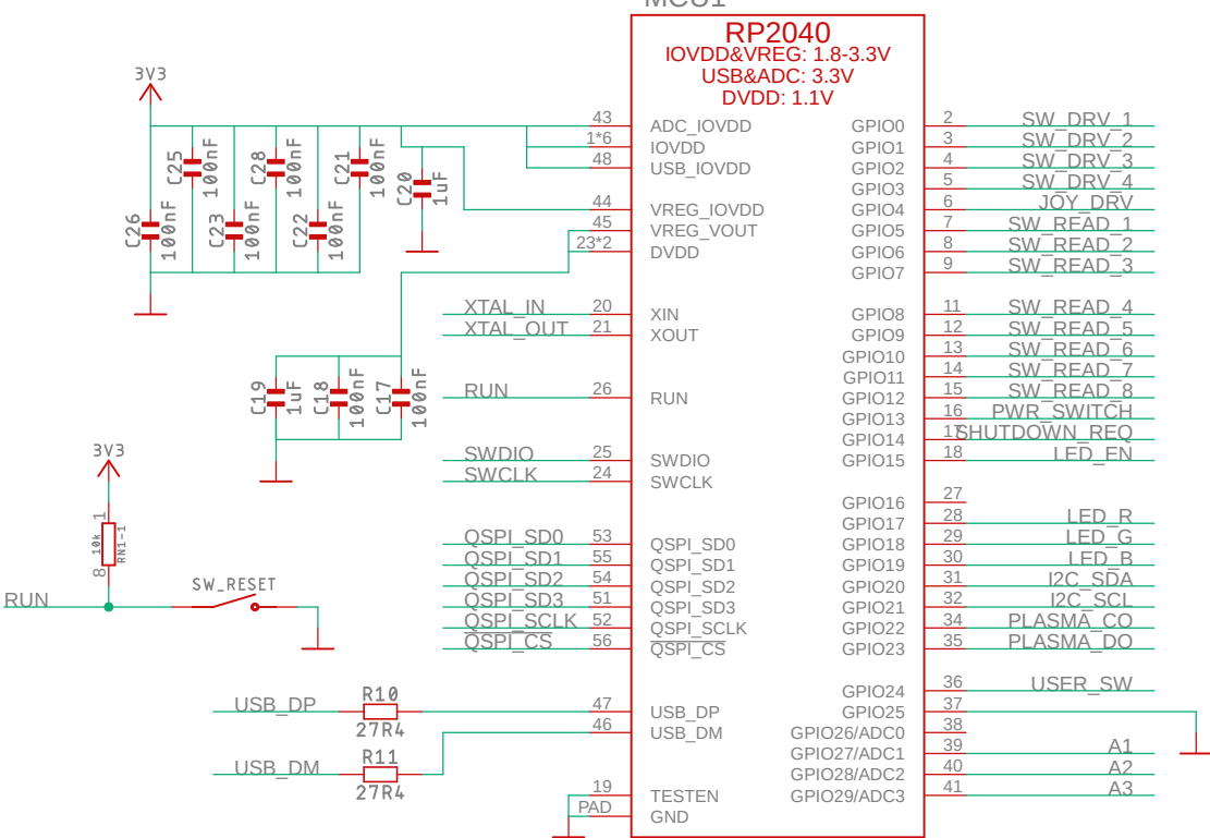
RP2040 MCU
