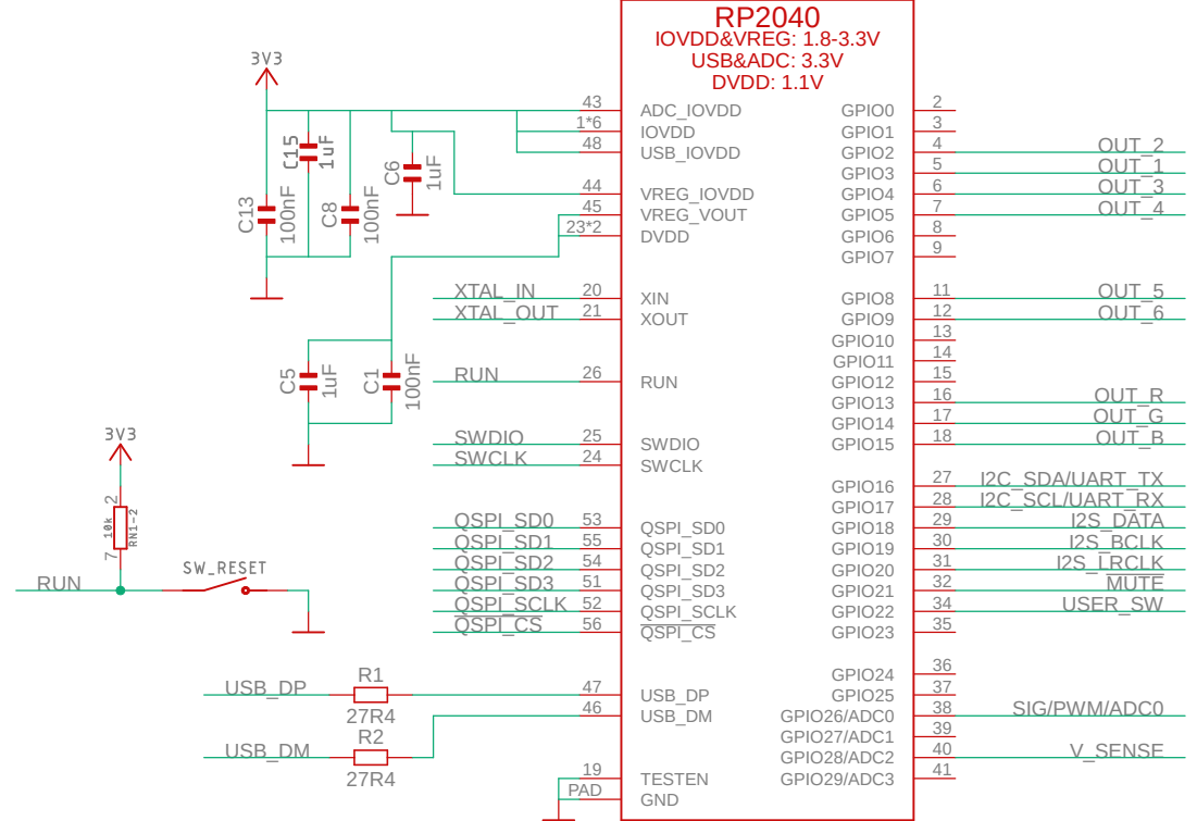
RP2040 MCU
