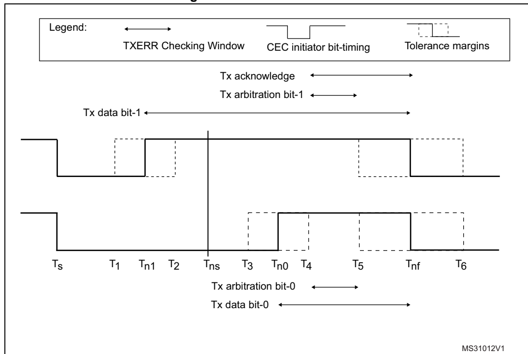
Figure 514. TXERR detection
