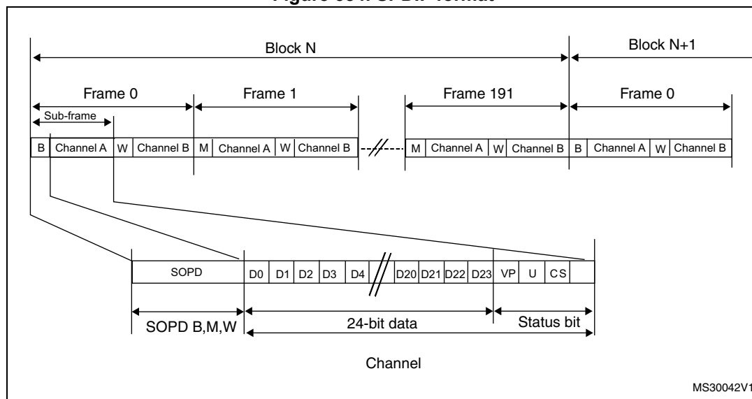
Figure 384. SPDIF format
