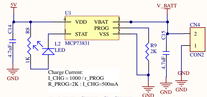
BATT CHRG CKT
