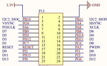
DCMI
