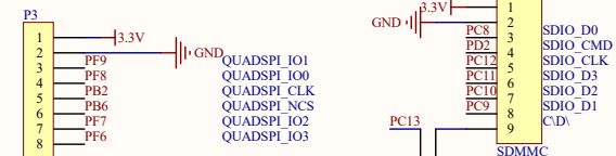
QUADSPI
