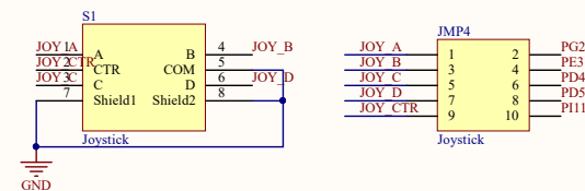
Joystick
