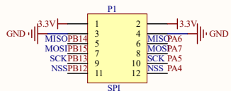
SPI2
