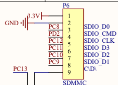
SDMMC
