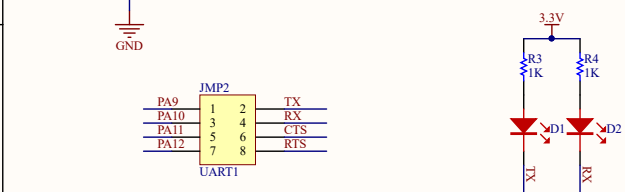
UART1
