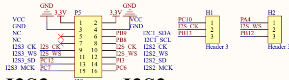
I2S3
