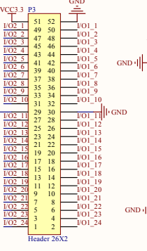
8I/Os_2
